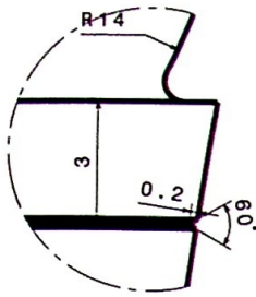
Détail K Echelle 10:1
